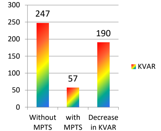
KVAR
