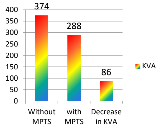
KVA Demand
